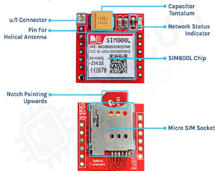
(Fig. 4.5 – SIM800L GSM Module)
