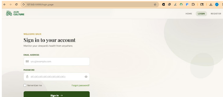
Fig 2. Login Module
